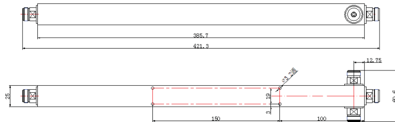
SP-03LX-43F-CC
